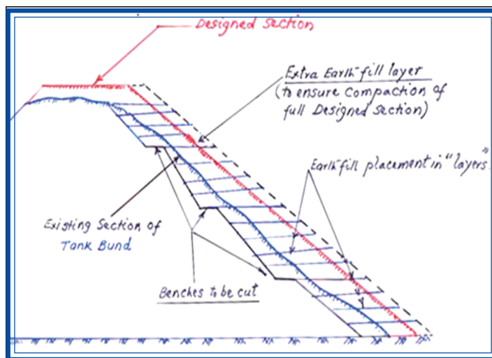
FIG: 5 EXTRA EARTH-FILL LAYER
