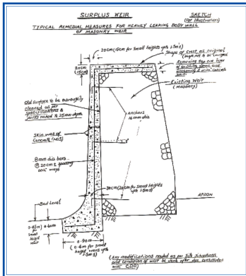
FIG: 15 SURPLUS WEIR
